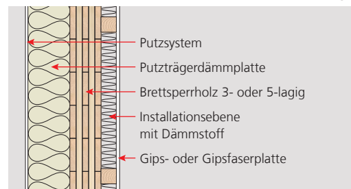
Beispiel Außenwand Holzmassivbau, mit Installationsebene, verputzt
