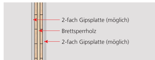
Beispiel Innenwand: Holzmassivbau, ohne Installationsebene, andere Oberfläche
