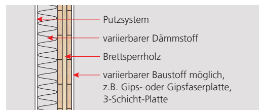
Beispiel Außenwand: Holzmassivbau, nicht hinterlüftet, ohne Installationsebene, verputzt
